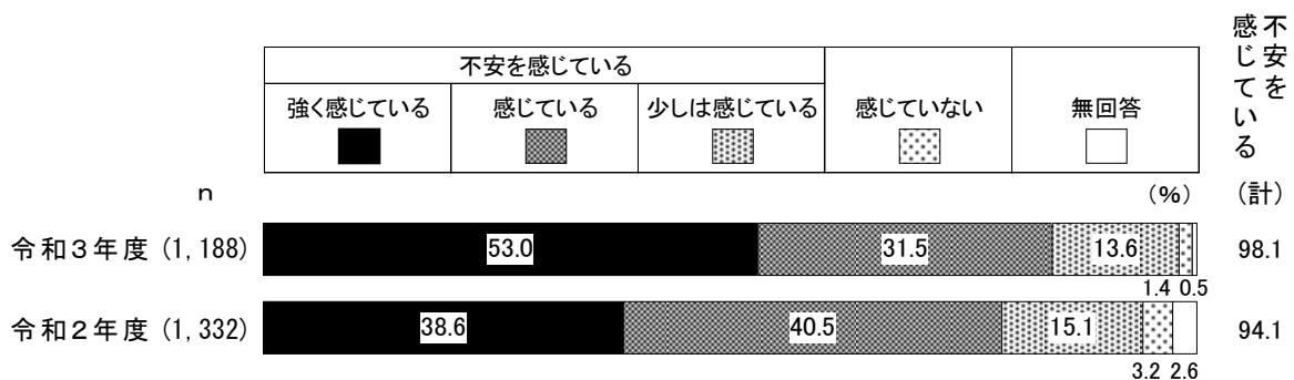
図2-2-2 新型コロナウイルス感染症に対して不安を感じる程度—過年度比較
