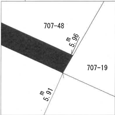
拡大図 縮尺 5分の1
