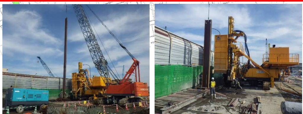
地中連続壁施工の様子
