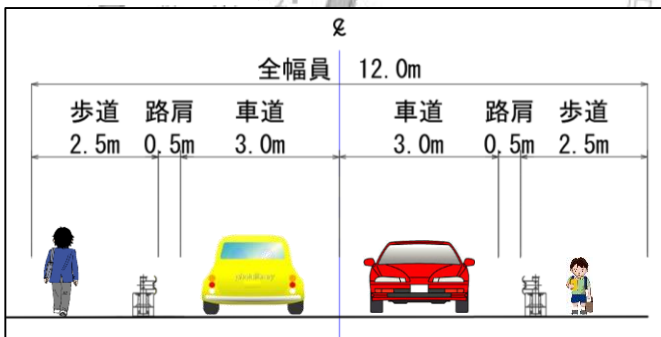
東映通り断面図
