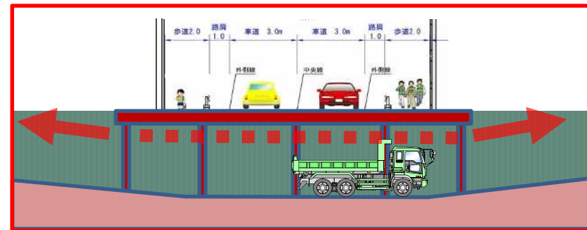
東映通り地下横断面図
