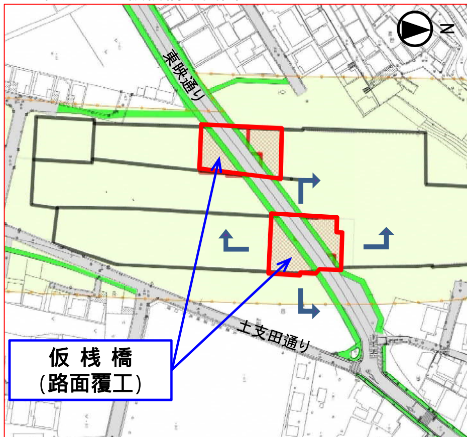
東映通りの仮棧橋平面図
