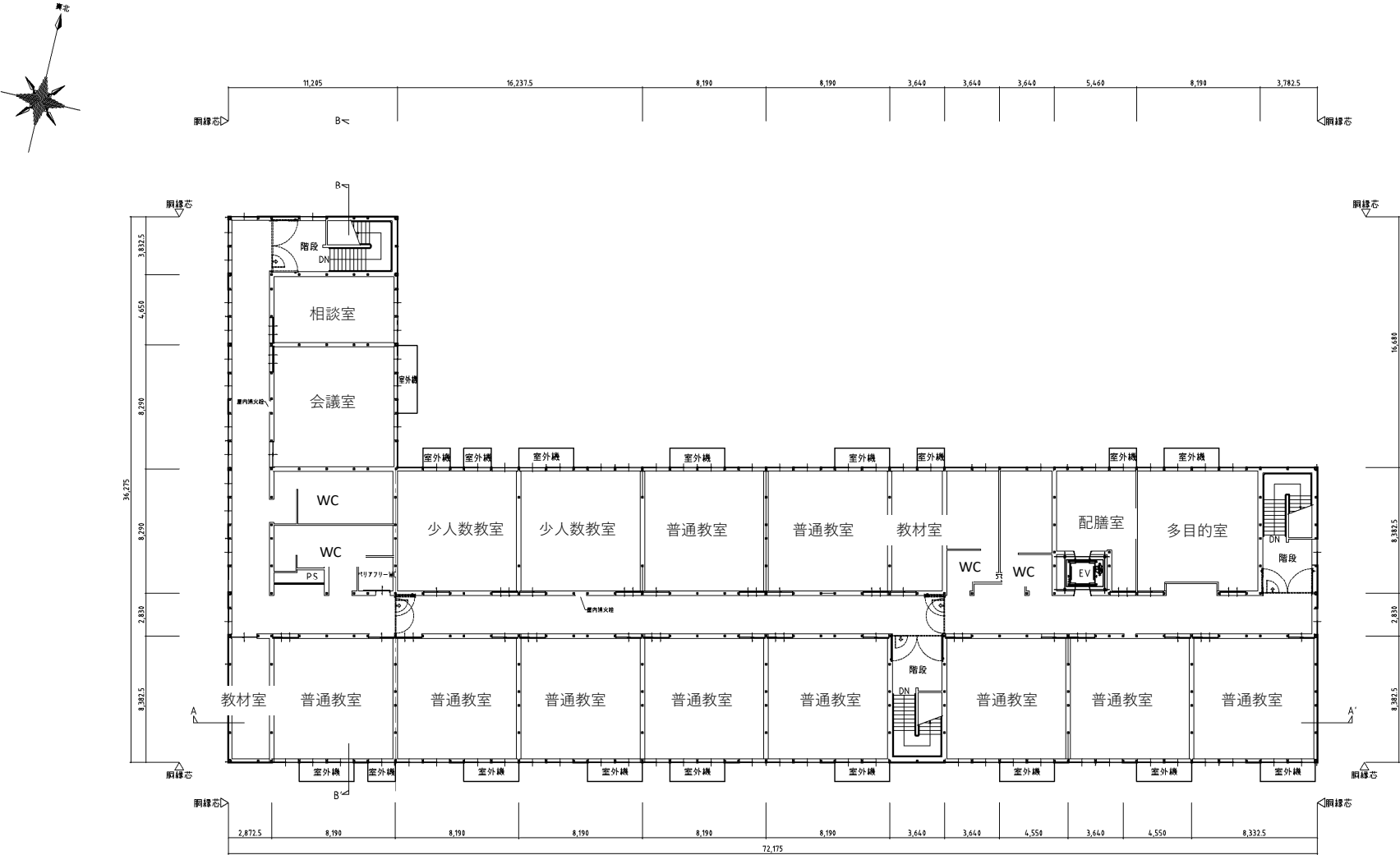
3 階平面図
