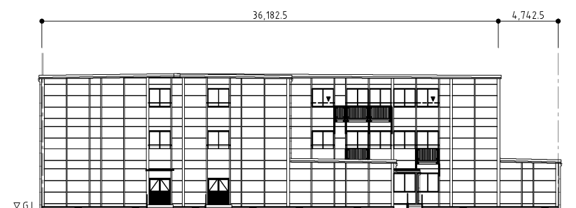
東側立面図
