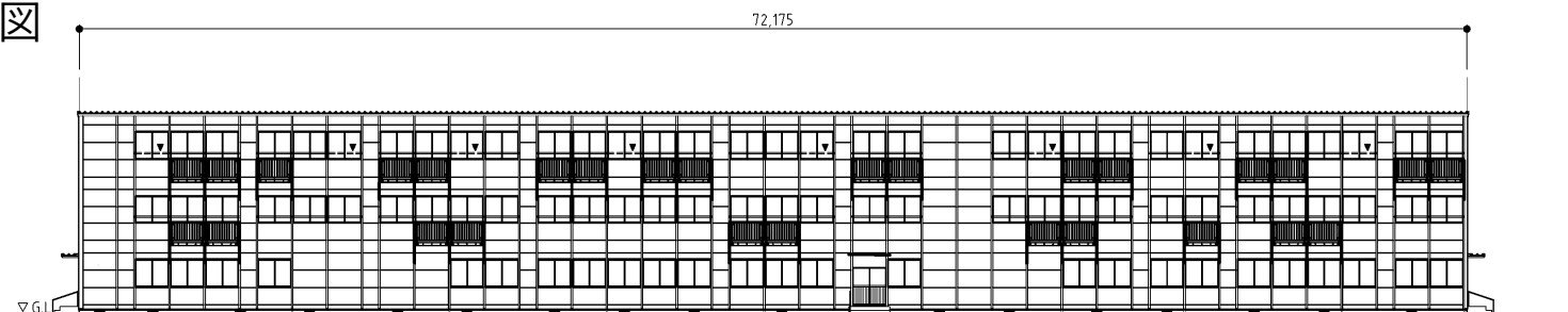
南側立面図
