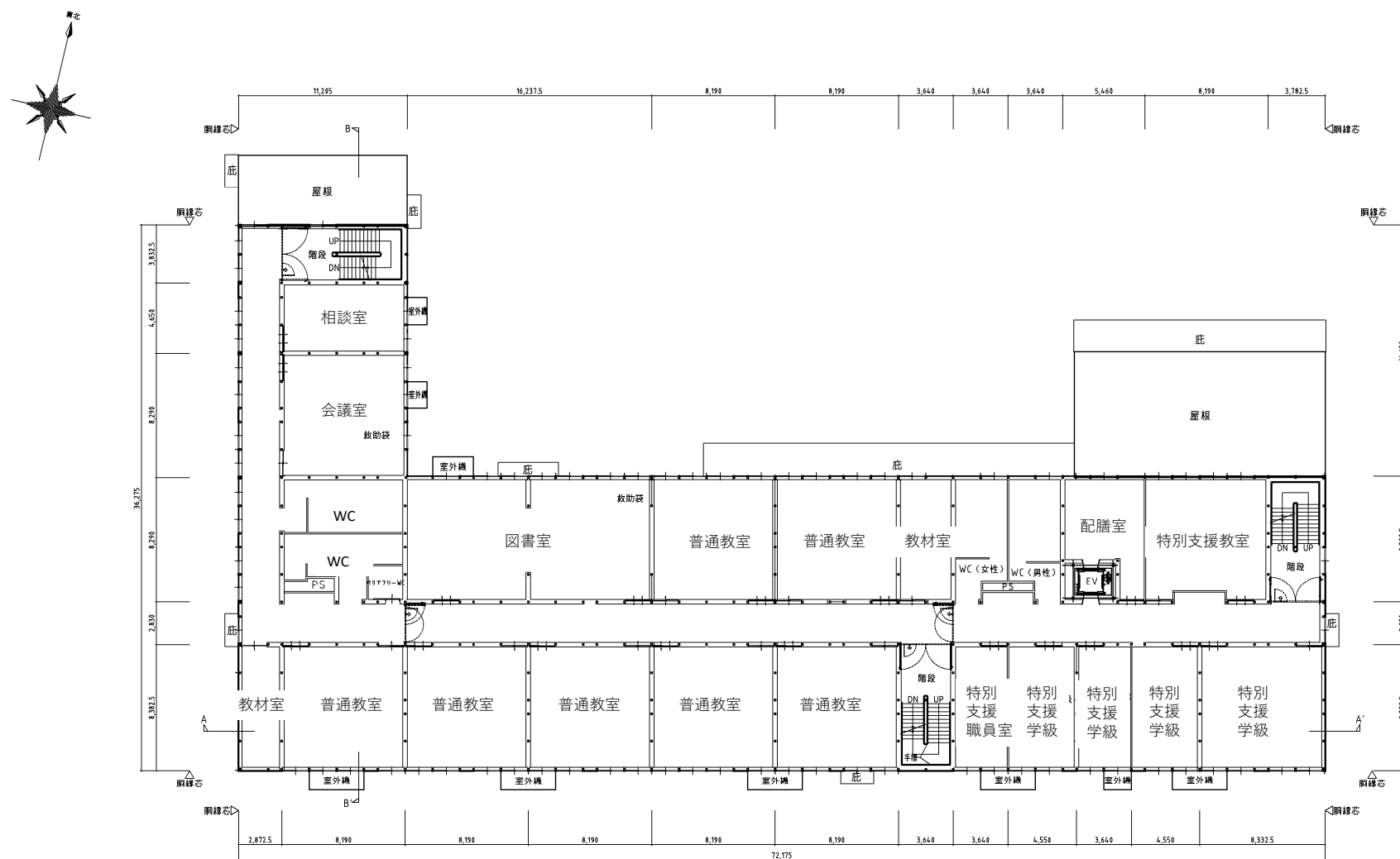
2 階平面図
