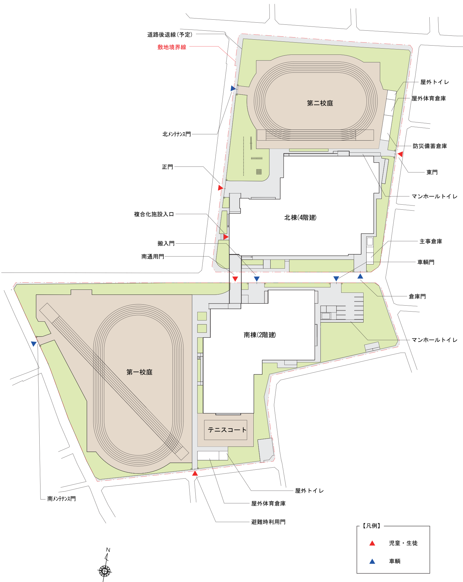
配置図
