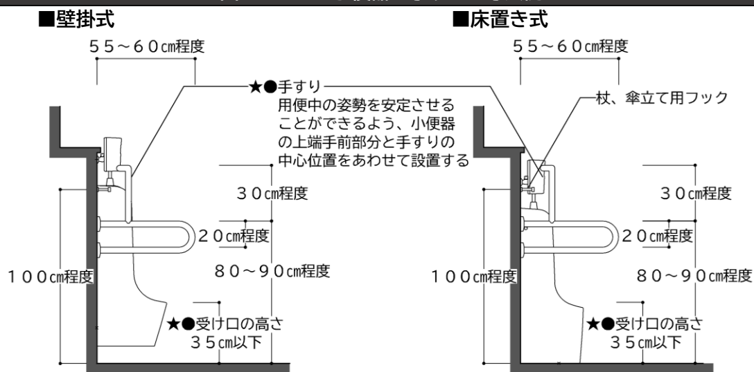
<図 I -8-12 小便器の手すりの寸法例>
