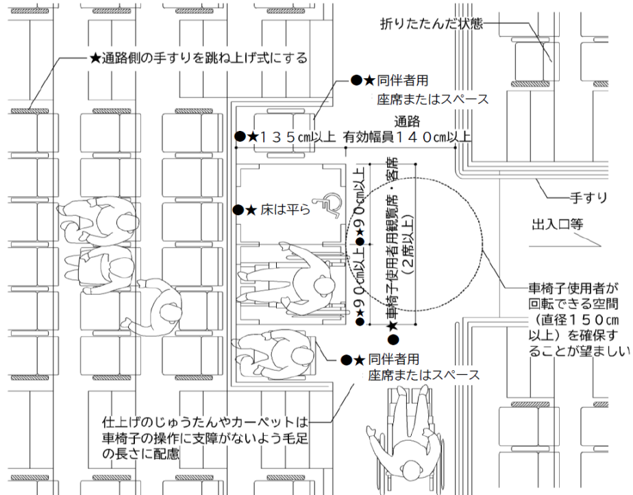
<図 I-11-1 観覧席・客席の例>
