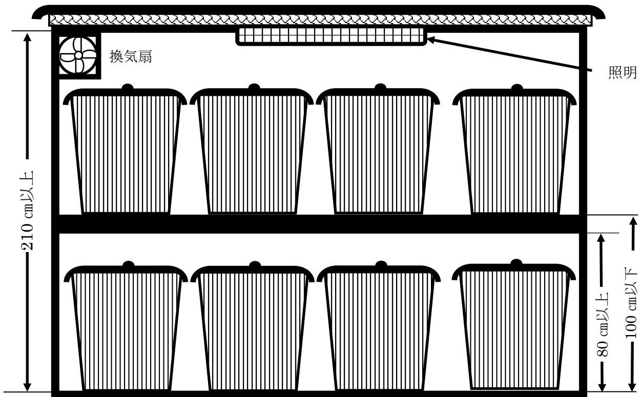
図2 廃棄物保管場所の断面図例
